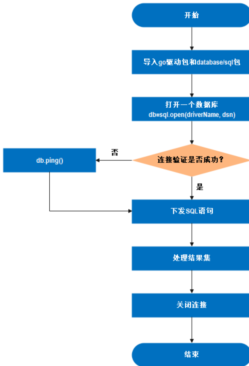
图 5-6 采用 Go 开发应用程序的流程图
