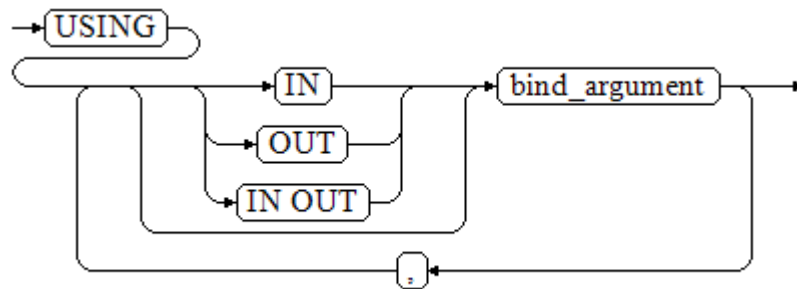
图 10-16 using_clause::=
