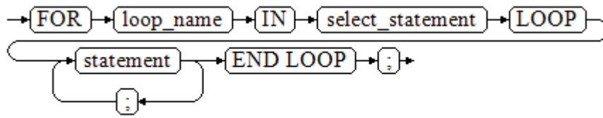
图 10-43 FOR_AS_loop::=
