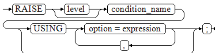
图 10-48 raise_condition::=
