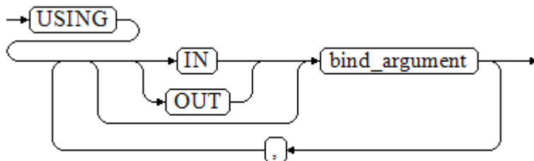
图 10-9 using_clause::=
