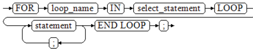
图 10-46 FOR_AS_loop::=
