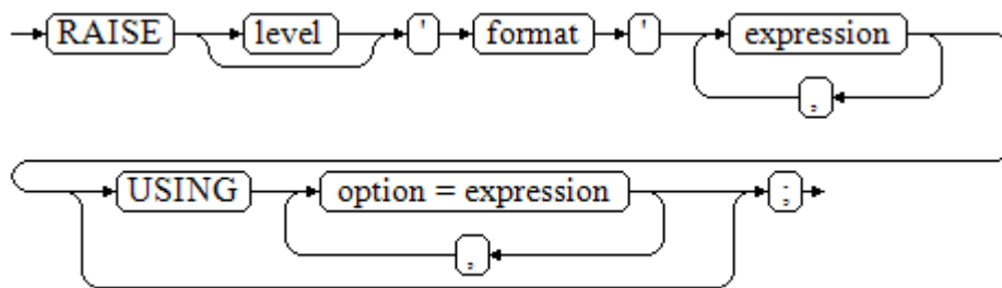
图 10-44 raise_format::=
