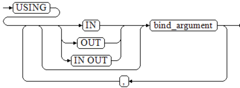
图 10-14 using_clause::=
