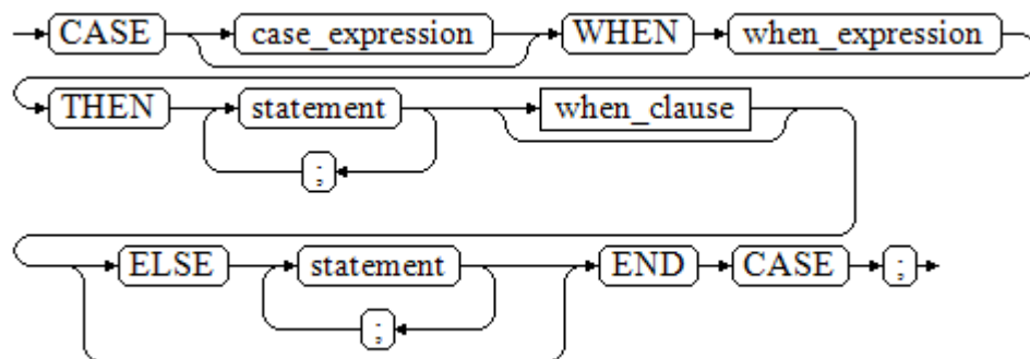
图 10-33 case_when::=
