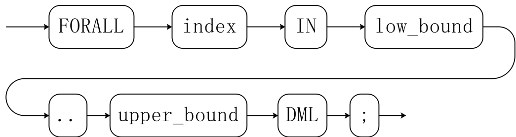
图 10-31 forall ::=
