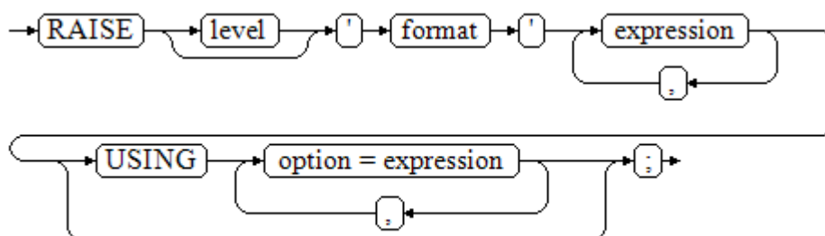
图 10-47 raise_format::=
