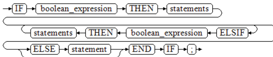
图 10-22 IF_THEN_ELSIF_ELSE::=
