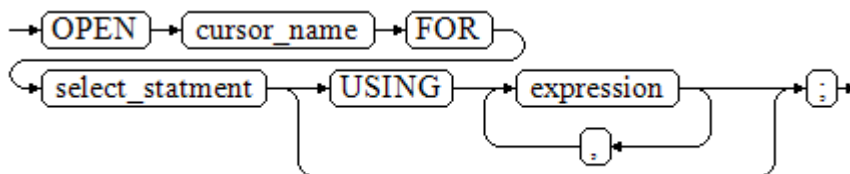
图 10-43 open_dynamic_cursor::=
